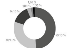
Verbleibender Energiemix
