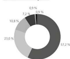
Verbleibender Energiemix
