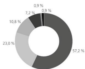
Verbleibender Energiemix
